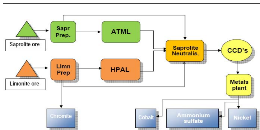
Fig. 1. Forenklet beskrivelse av behandlingsprosessen for Mindoro Nickel lateritt
